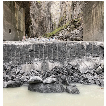
Rückbau einer Betonsperre in der Schlucht
